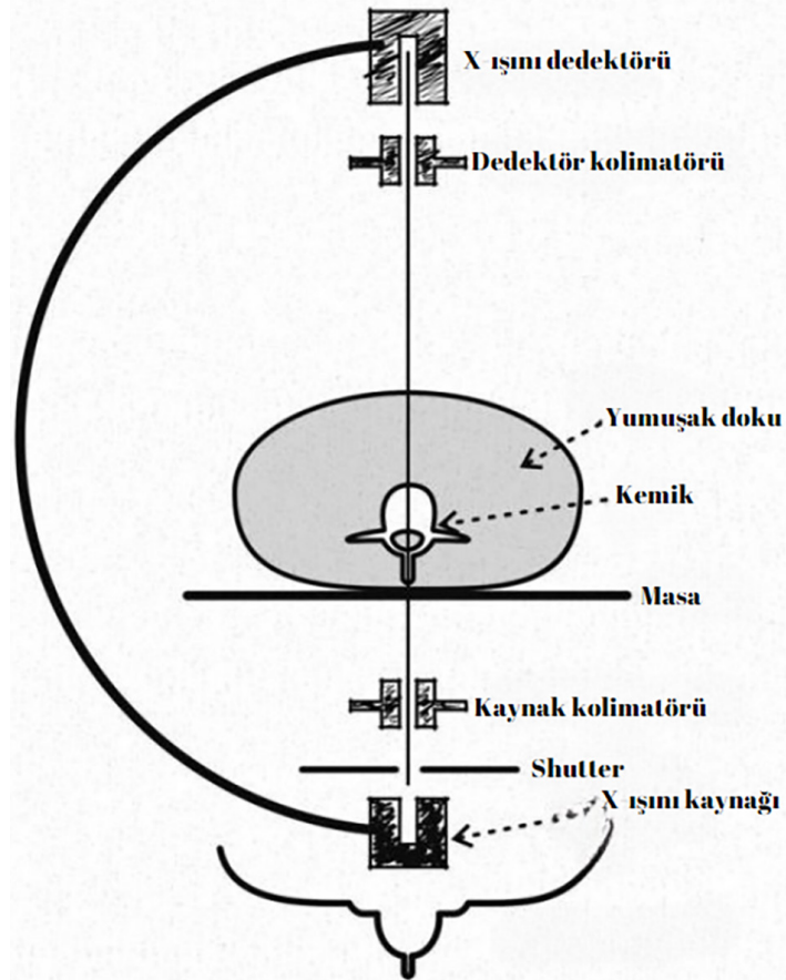
Resim 8. DXA sisteminin bileşenlerini gösteren şematik diyagram [24].
